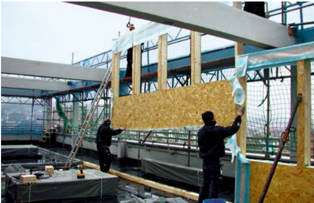
Erweiterung durch Überbauung der Dachterrasse im 7. Obergeschoss für zwei Besprechungsräume und Büros im Jahr 2009.
